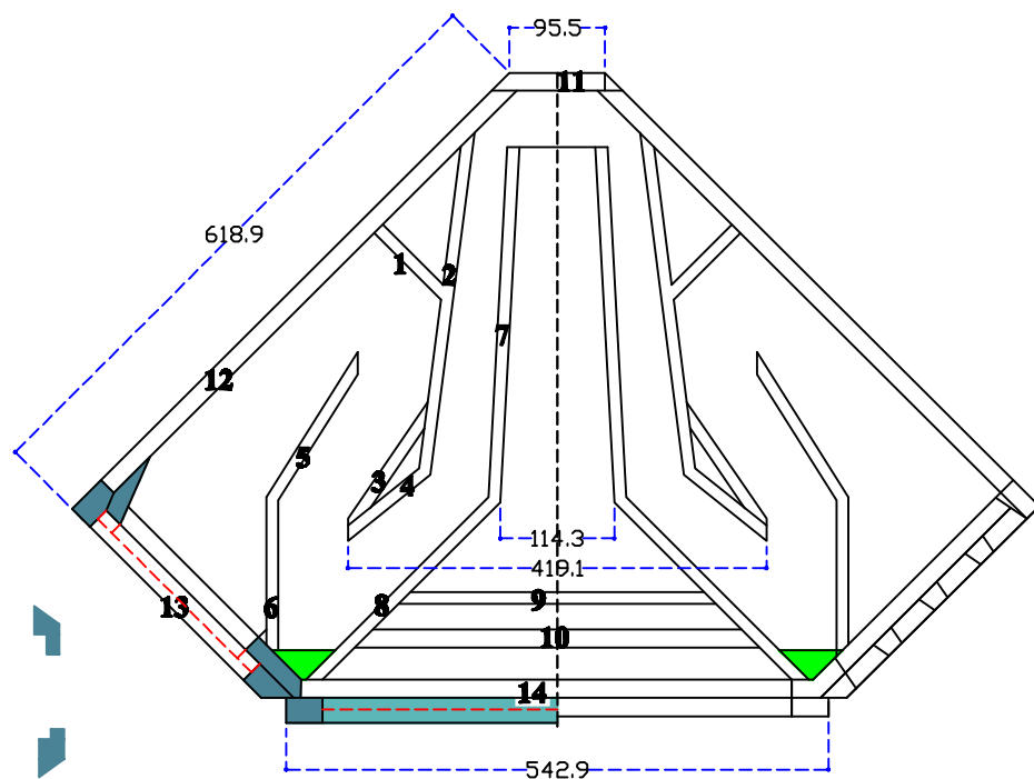
Thùng loa GRF Horn Plywood Người Vẽ : Trung_Hiếu 06/2011
