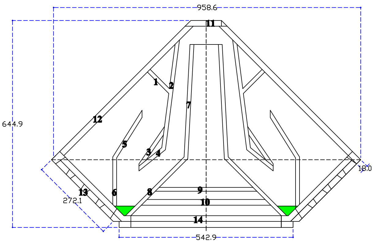
Thùng loa GRF Horn Plywood Người Vẽ : Trung_Hiếu 06/2011
