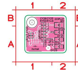
PY46 PWB A
